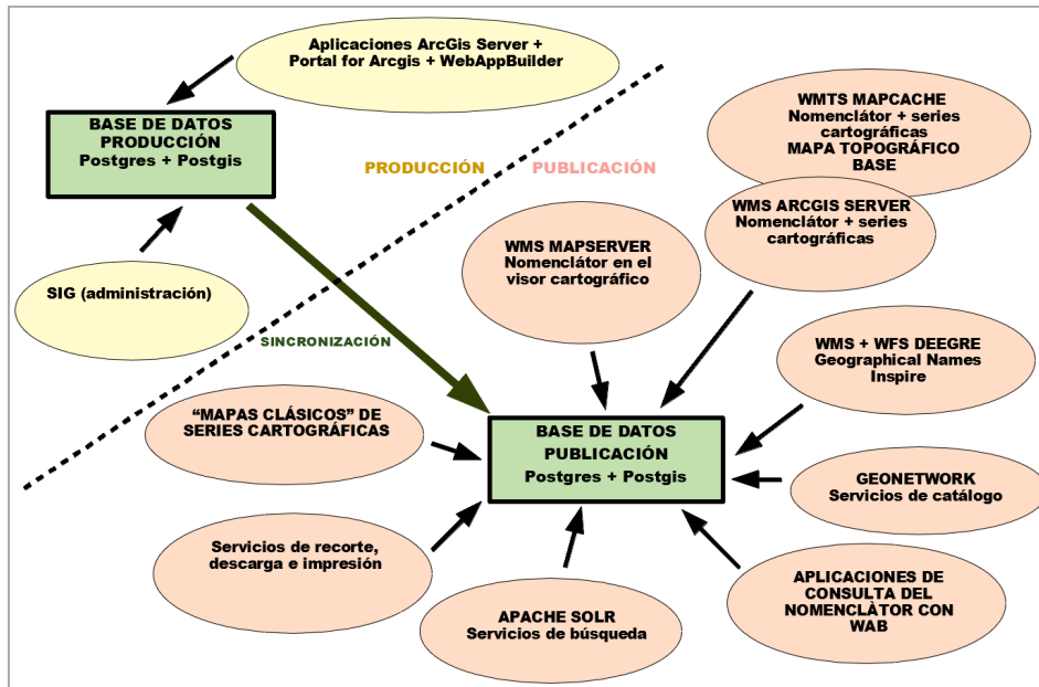
Figura 6: Arquitectura Producción - Publicación del NTV
